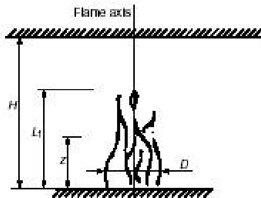
Fig. 6.3: Model van een plaatselijke brand, waarvan de vlammen niet tot het plafond reiken
