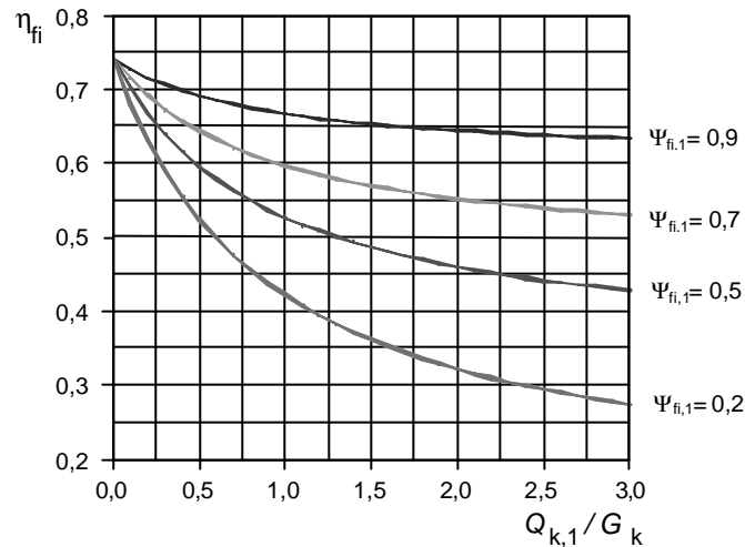
Fig. 7.1: De reductiefactor \eta_{fi} als functie van de verhouding Q_{k,1} / G_k voor verschillende waarden van de combinatiefactor \Psi_{fi,1}
